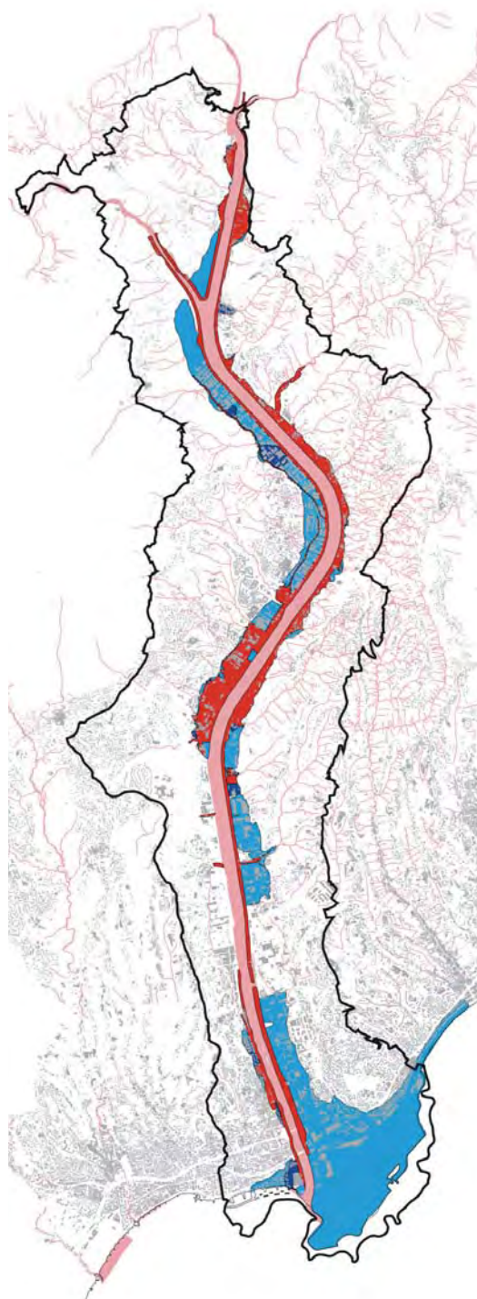
prospective du PPRI une fois PAPI réalisé
